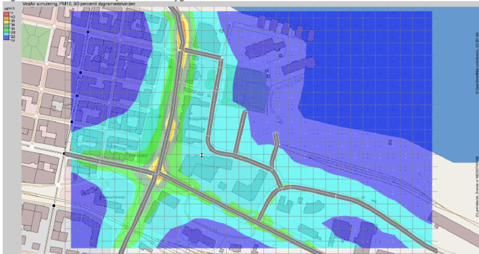
Figur 11. Partiklar som 90-percentil för dygnsmedelvärde år 2015
