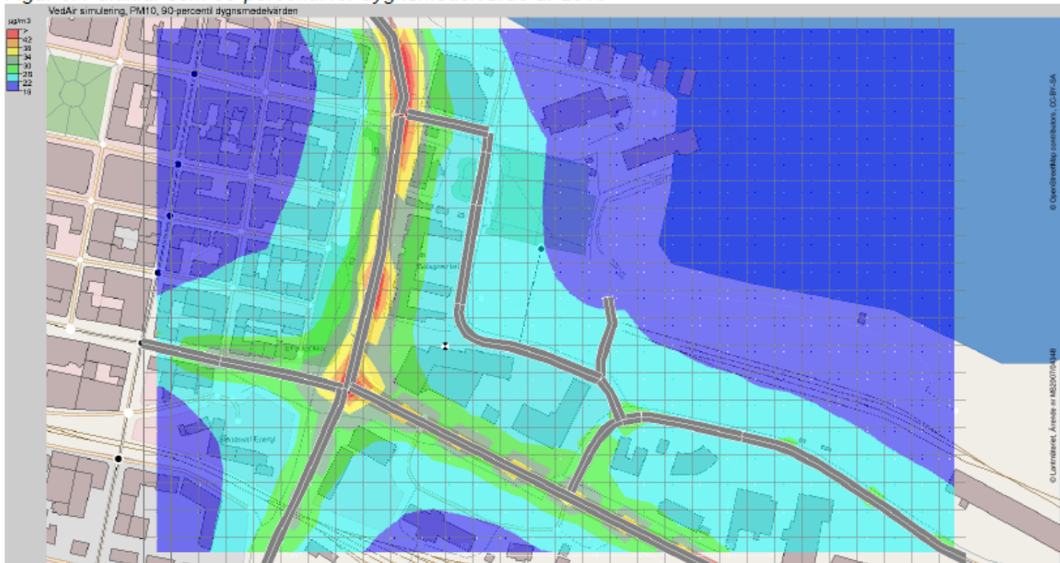
Figur 6. Partiklar som 90-percentil för dygnsmedelvärde år 2010
